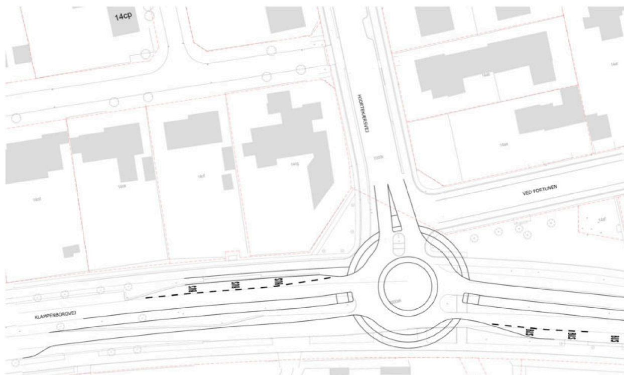
Figur 6: Løsningsforslag, hvor krydset ombygges til en rundkørsel.
