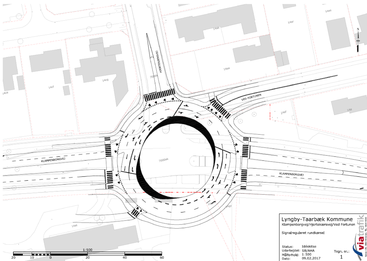
Figur 2: Forslag til udformning af rundkørslen.
